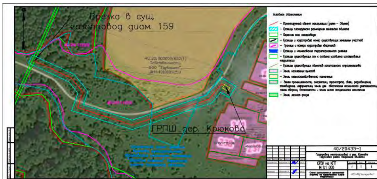
Рисунок 3.1 – Обзорная схема участка строительства
